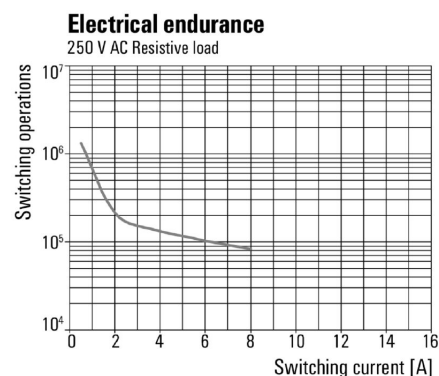
Elektrická životnost 250 V AC odporová zátěž
