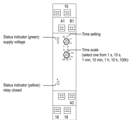
Detailní výkres
