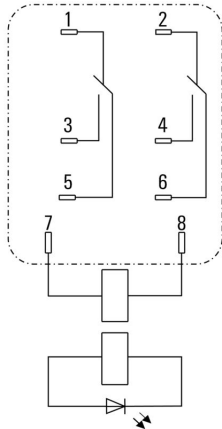
Pohled na piny ze spodní strany
