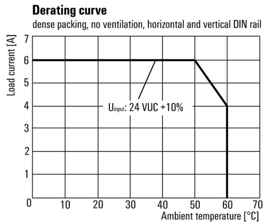
Křivka odlehčení
