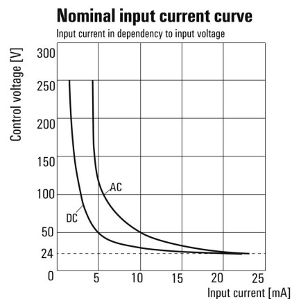
Vstupní proud v závislosti na vstupním napětí
