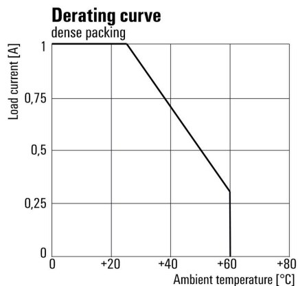
Křivka odlehčení
