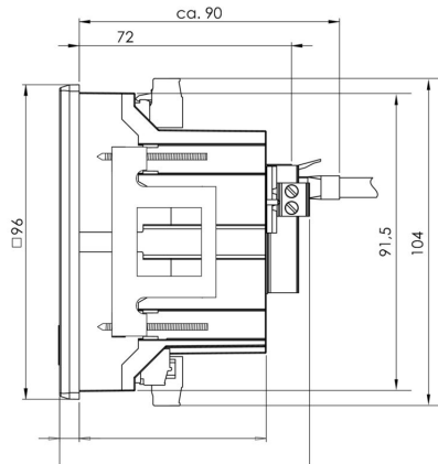
Rozměrový výkres
