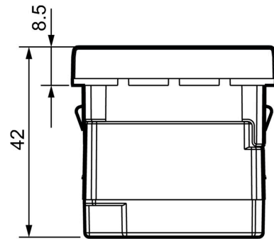
Rozměrový výkres
