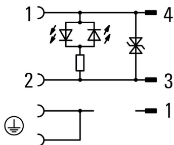
Schéma připojení
