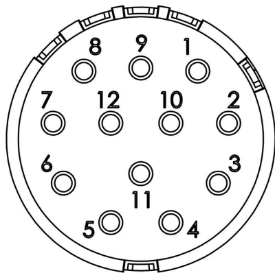
Rozměrový výkres
