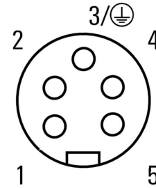
Socket
