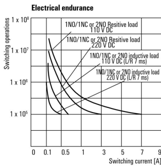
Elektrická životnost
