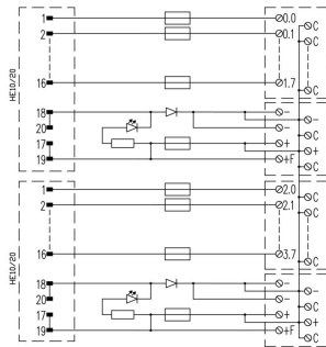
接线图适用于带 LED 的规格。
