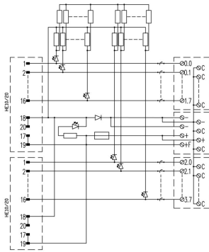
接线图适用于带 LED 的规格。
