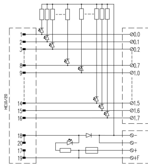
接线图适用于带 LED 的规格。
