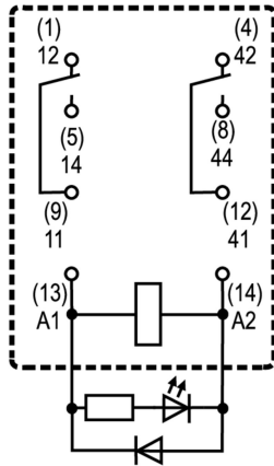
插针仰视图
