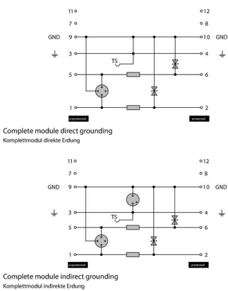
Kompletmodul
