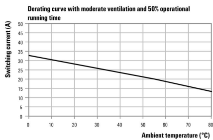
直流负载极限曲线
