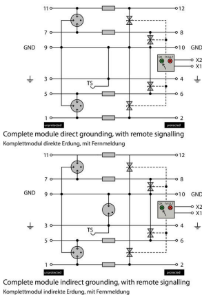
Kompletmodul
