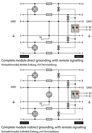
Kompletmodul
