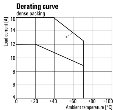
电流温度曲线 继电器与底座搭配
