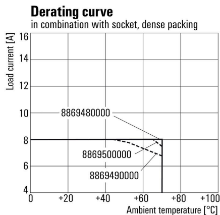
电流温度曲线 继电器与底座搭配
