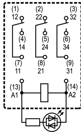
插针仰视图
