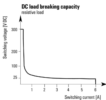
直流负载极限曲线
