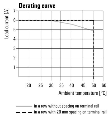
电流温度曲线
