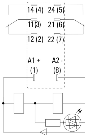
插针仰视图
