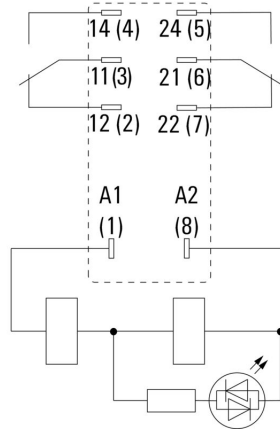
插针仰视图
