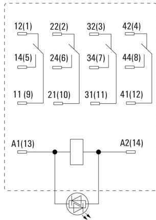
插针仰视图
