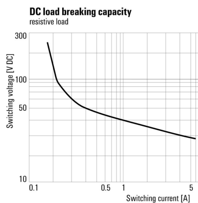
直流负载极限曲线 阻性负载
