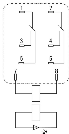
插针仰视图
