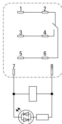
插针仰视图
