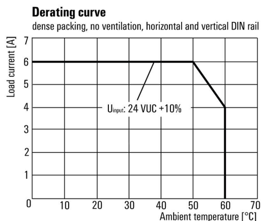
电流温度曲线
