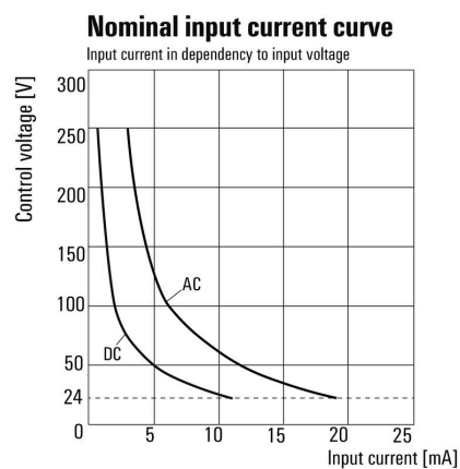
输入电流依赖于输入电压
