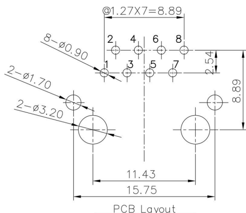
电路板布局
