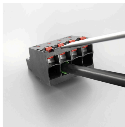
Quick wiring
