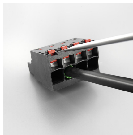
Quick wiring
