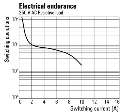
电气寿命
