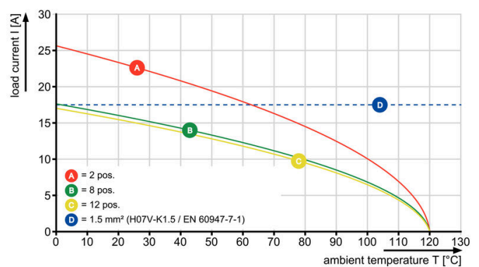
BCL-SMT 3.81/./180 - SCZ 3.81/./180
