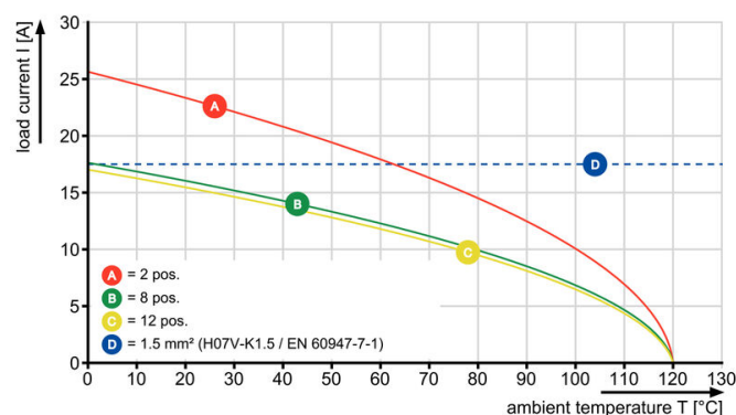
BCL-SMT 3.81/./180 - SCZ 3.81/./180
