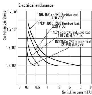
电气寿命
